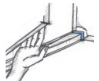
FONDI PENSILE CON PRESA MANIGLIA WALL UNIT BOTTOM PANELS WITH GRIP EDGES
